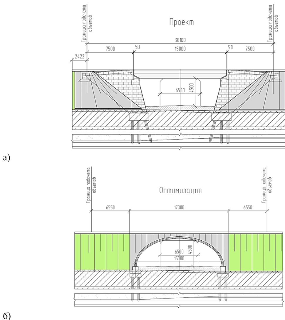
Рис. 1. Варианты решений: а) - предусмотренное проектом; б) - предложенное независимым консультантом в результате проведения ТЦА
